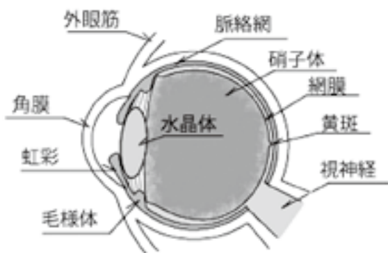
眼の構造
