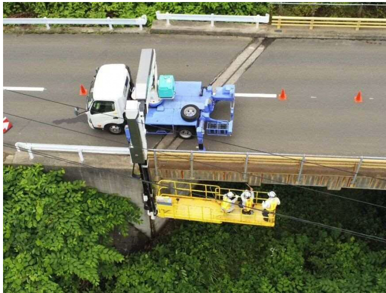
従来の点検方法（橋梁点検車）
